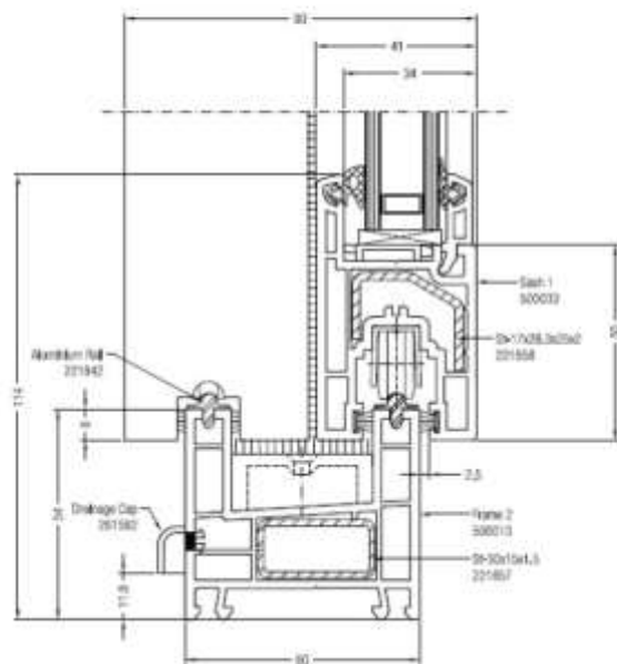
Sezione nodo 2 ante scorrevoli finestra ( vista laterale )
