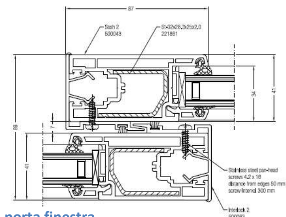
Sezione nodo 2 ante scorrevoli porta finestra ( vista da sopra )
