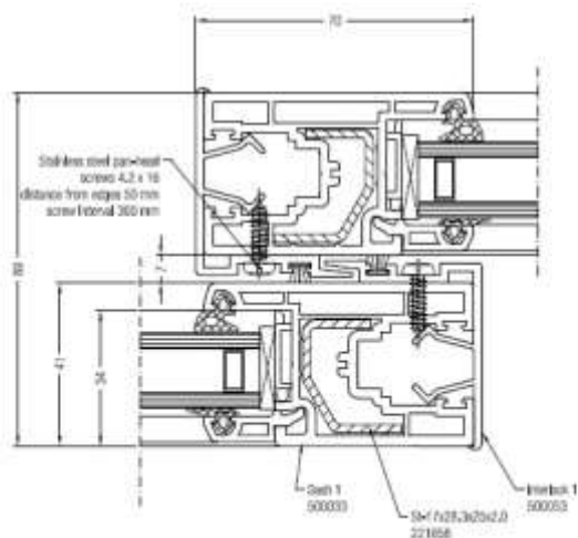
Sezione nodo 2 ante scorrevoli porta finestra ( vista da sopra )
