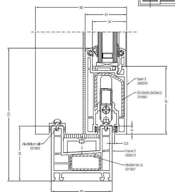
Sezione nodo 2 ante scorrevoli porta finestra ( vista laterale )
